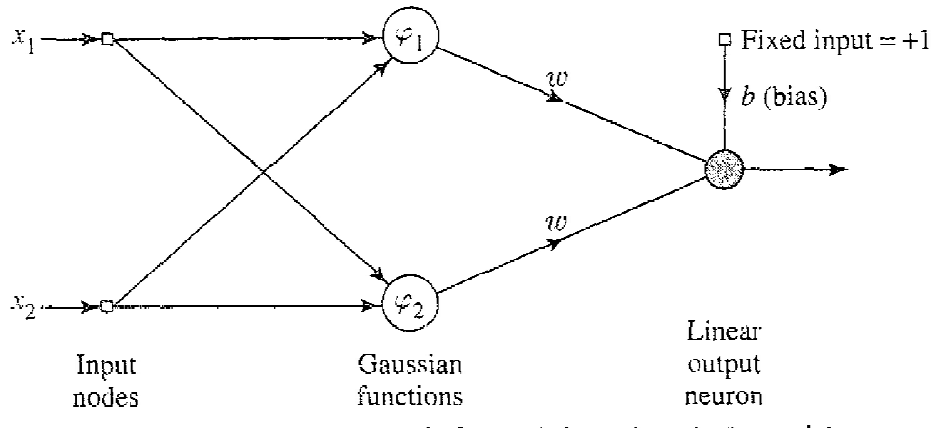
Figure 2: Rede Neural para resolução do problema do XOR [1].
