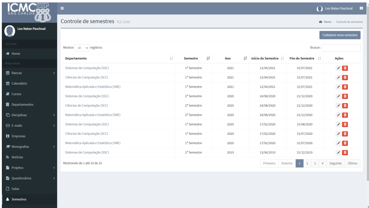
Figura 2.4. Interface para gerenciamento de semestres
