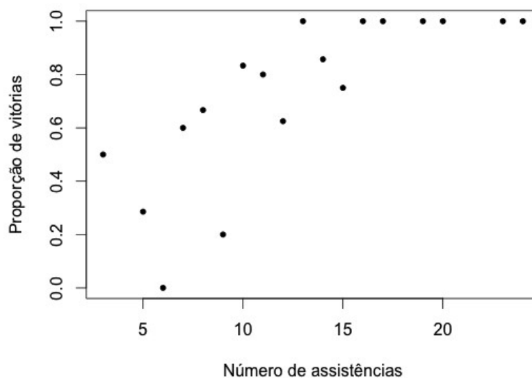
Figura 1. Proporção de vitórias do Boston Celtics versus número de assistências de Rajon Rondo.
